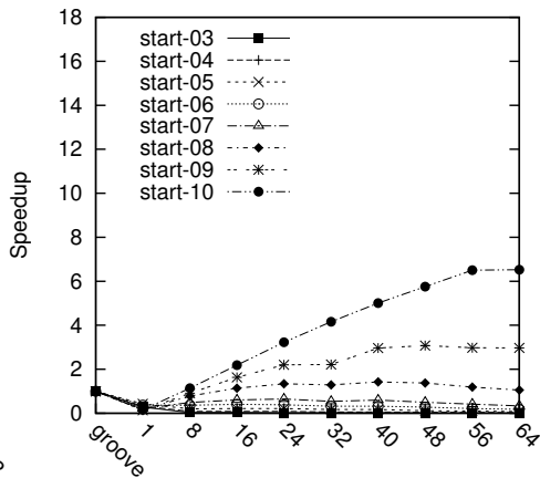
(d) unflagged-platoon, enc_N . Speedup compared to GROOVE.
