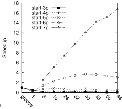
(d) 1e, enc_N . Speedup compared to GROOVE.
